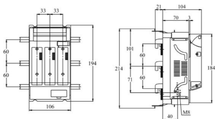
尺寸图/ Dimensions drawings 00型/ Size 00
