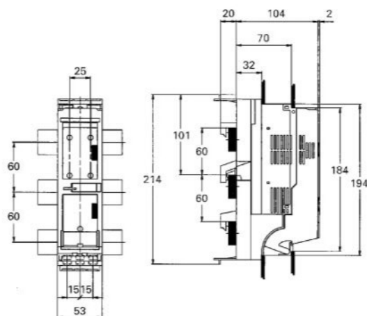
尺寸图/ Dimensions drawings 00型/ Size 00
