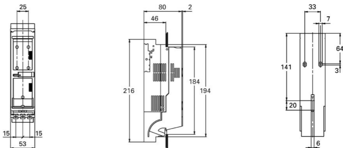
尺寸图/ Dimensions drawings 00型/ Size 00
