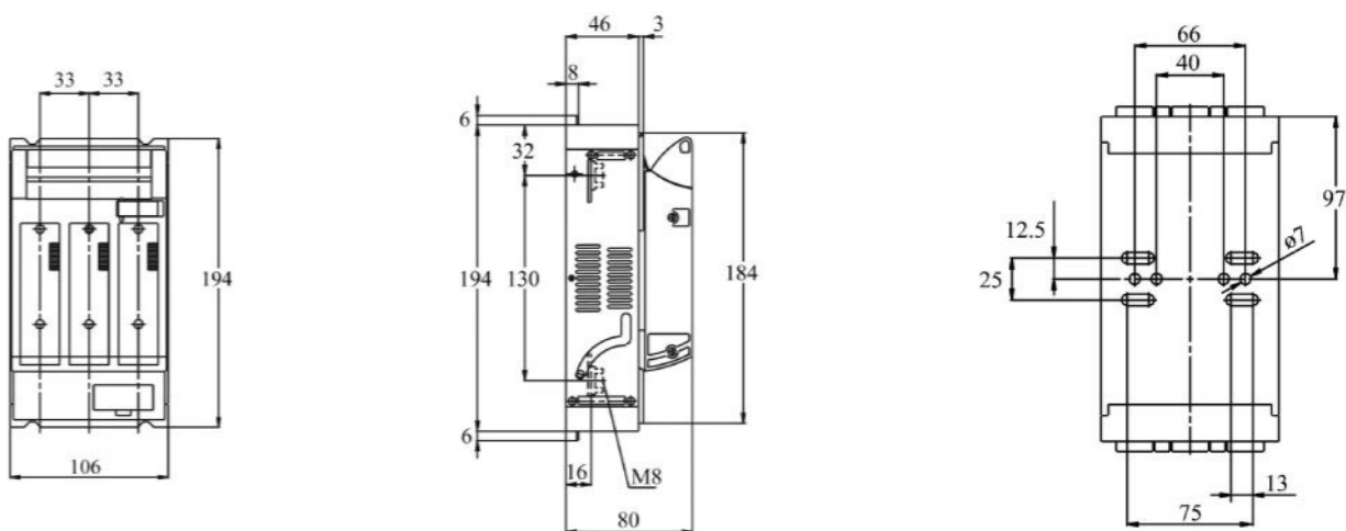
尺寸图/ Dimensions drawings 00型/ Size 00
